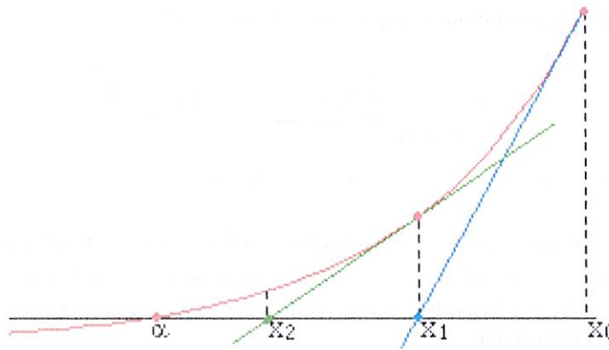
FIGURE 1 – Illustration géométrique de la méthode de Newton sur une fonction convexe.
